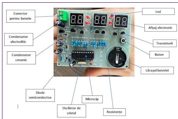
Montaj ceas digital
