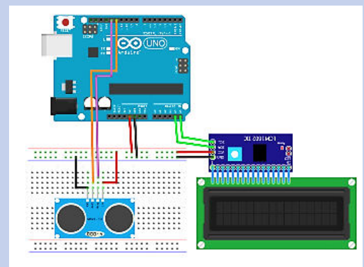
Montaj pentru măsurarea distanței ultrasunete și afișaj numeric
